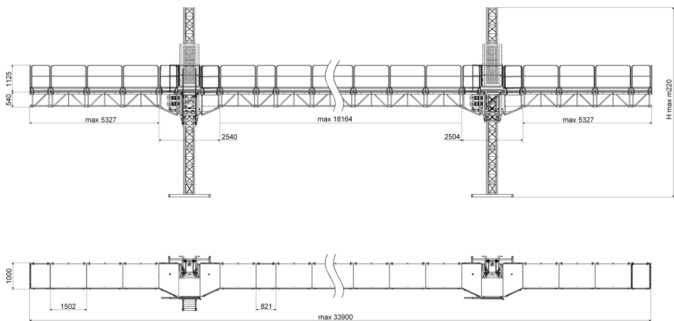
PLATFORMA MONOCOLOANA P 40/1 ОДНОМАЧТОВАЯ ПЛАТФОРМА P 40/13
